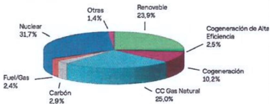
Figura 4: Mix eléctrico.
